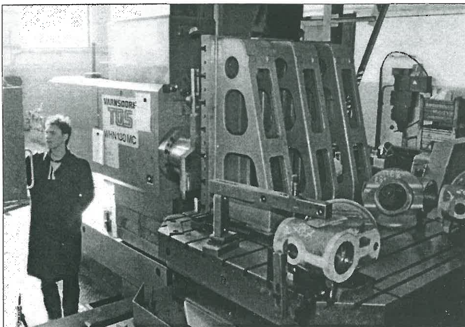
Nově vybudované pracoviště WHN 130 MC v plném provozu
