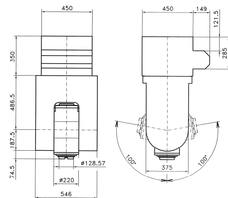
Общий вид головки
